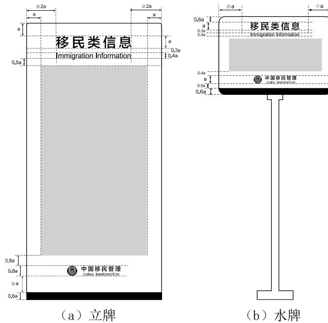
图22 口岸信息提示牌（立牌、水牌）标志规格
