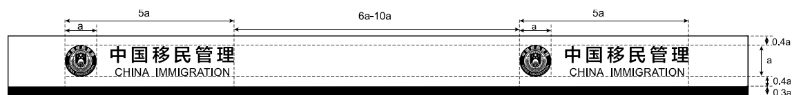
图14 执勤设施腰线标志规格
