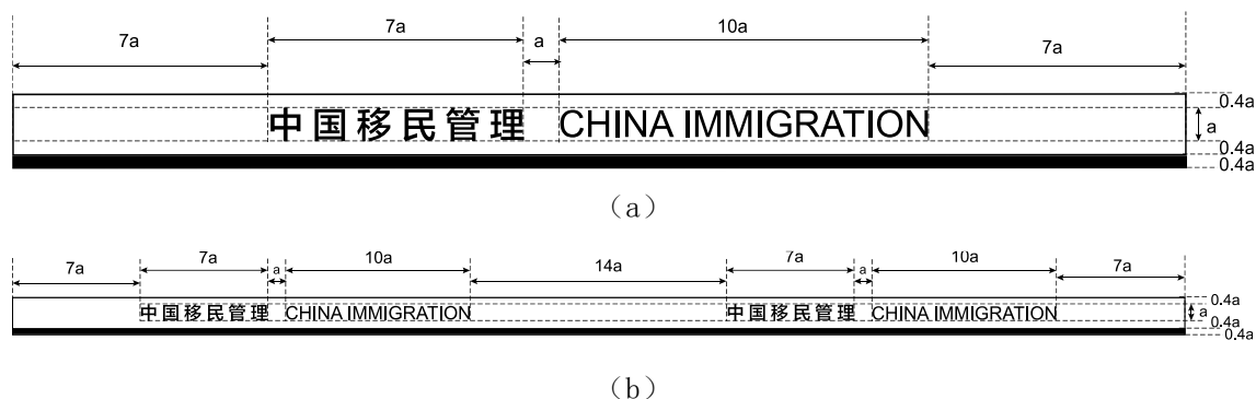
图12 软隔离设施标志规格
