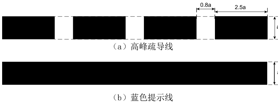
图25 高峰疏导线标志和蓝色提示线标志规格
