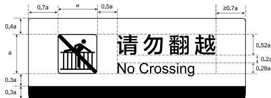
图27 请勿停留、请勿使用手机、请勿翻越、请勿抛物、请勿通行和请勿入内 6 个劝阻标志规格
