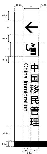
图31 导向标志纵向布置规格
