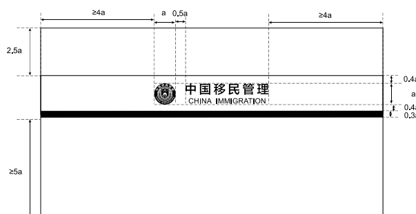
图13 硬隔离设施标志规格
