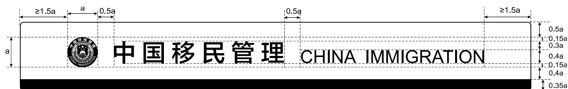
图15 室外执勤设施门头（横标）标志规格
