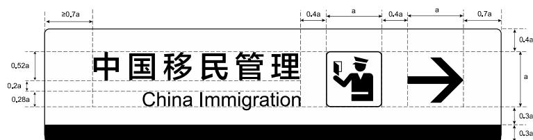
图30 向右前、向右和向右下 3 个导向标志横向布置规格
