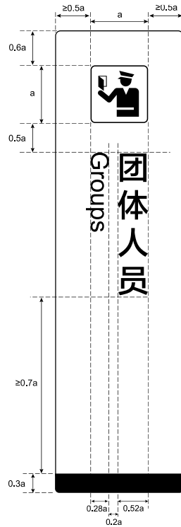
图3 纵向布置的标志规格样式
