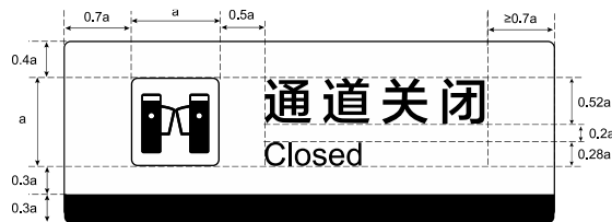
图24 通道关闭标志规格
