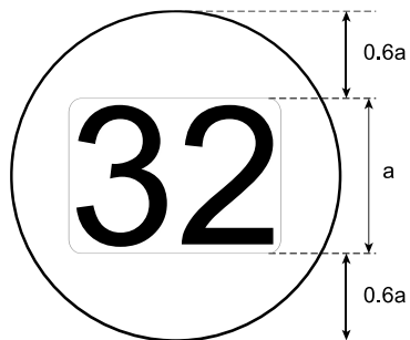
图7 通道号规格
