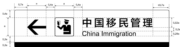
图29 向前（上）、向左前、向左、向左下、掉头、上楼和下楼 7 个导向标志横向布置规格
