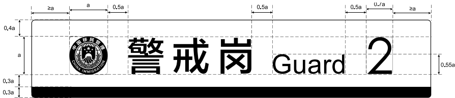
图11 警戒岗（超长）和监护岗（超长）2个设施标志规格
